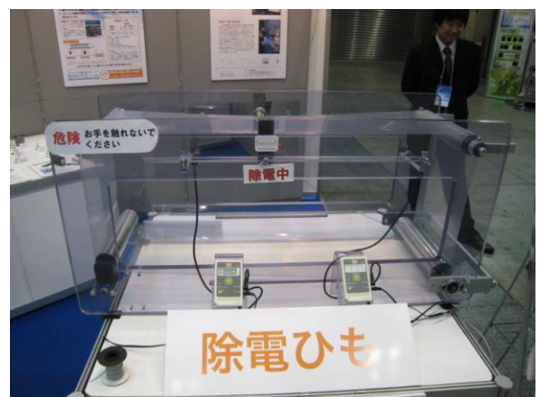
連続式フィルム回転デモ装置
